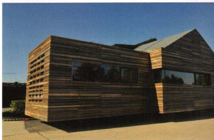
Le bâtiment de bureaux magnifique, entièrement réalisé en ossature bois et isolé avec de la laine de mouton.
